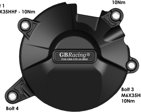
Bolt 4 M6X35HHF - 10Nm
